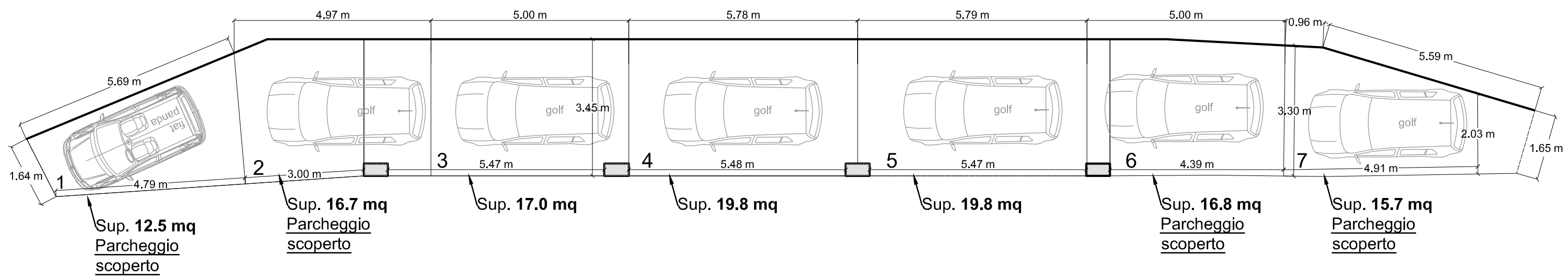
Planimetria stato di progetto con indicazione della nuova numerazione, delle dimensioni e delle superfici dei posti auto - Scala 1:100
